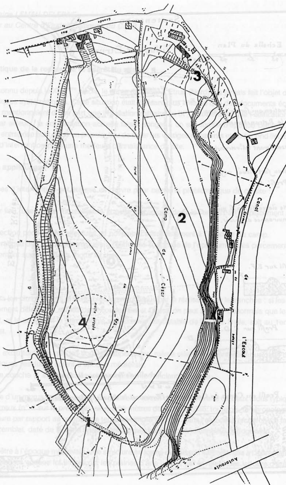
Camp de César (Etrun) : 1991, zones d'intervention
