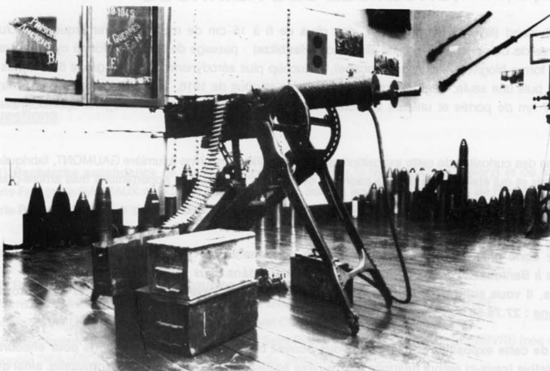
Mitrailleuse lourde MAXIM 08 (Mashinengewehr MG 08). Poids : 26 kg 450. Calibre : 7,92 millimètres. Refroidissement par eau. Cadence de tir : 300 à 400 coups/minutes. Vitesse initiale : 892 mètres/seconde.
