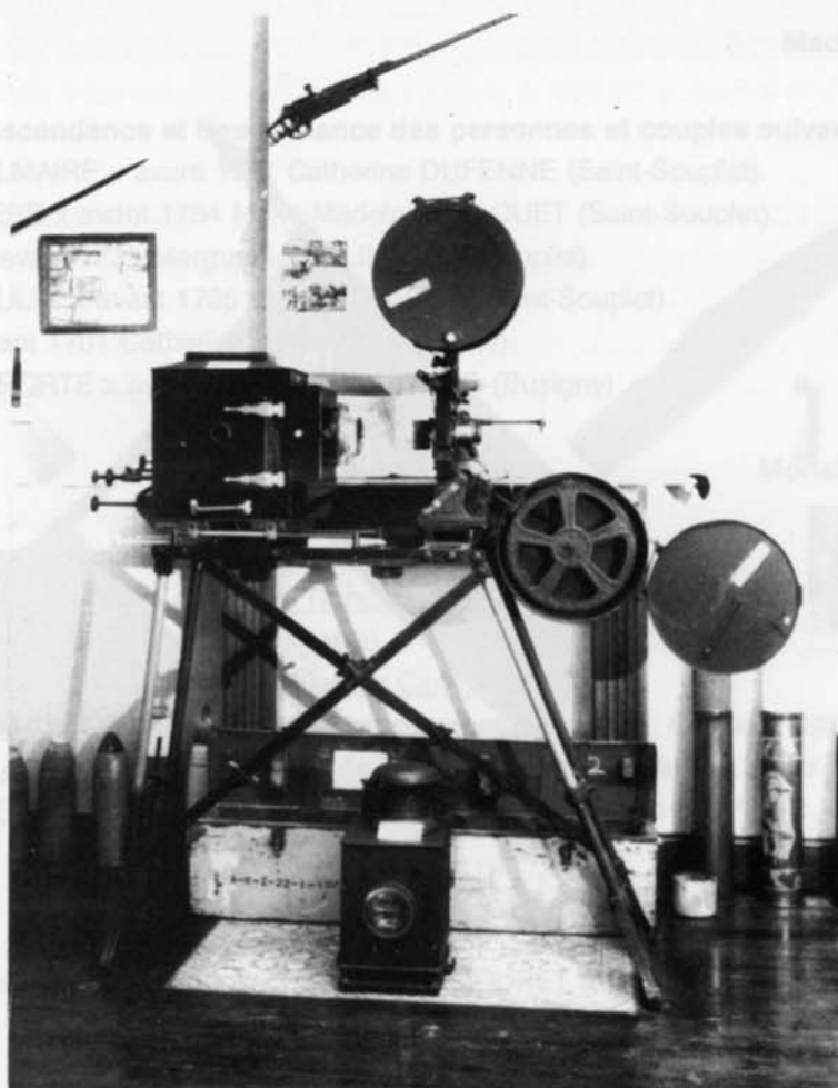
Machine à lumière GAUMONT fabriquée en 1907 à Paris, utilisée dans le cadre du cinéma des Armées
